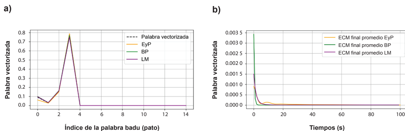
■ Figura 6. Comparación del aprendizaje (a) de la palabra badu-pato y (b) sus respectivos errores cuadráticos medios (ECM) iniciales.
